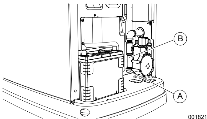
Figura 4-7. Limpieza de la trampa para sedimentos
